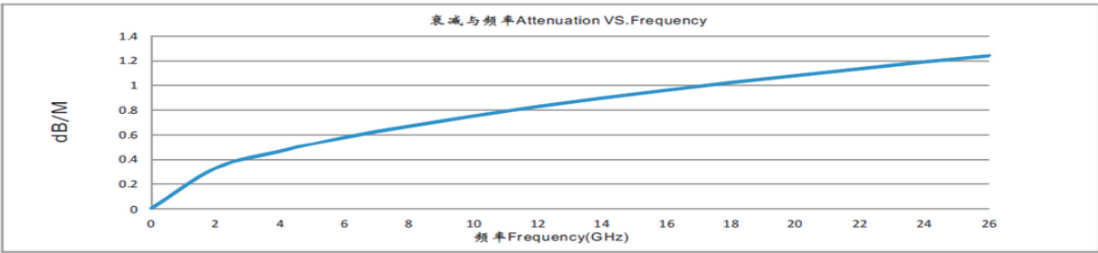
电缆衰减/Cable Attenuation 典型值@ +25 环境温度 Nominal Values @+25 Ambient Temperature
